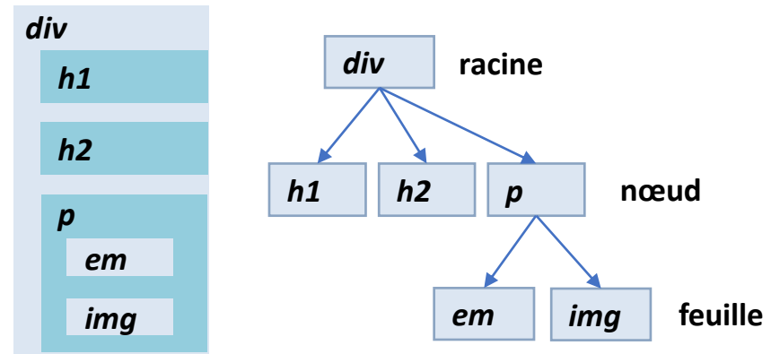
Figure 10 : Encapsulation des balises HTML
