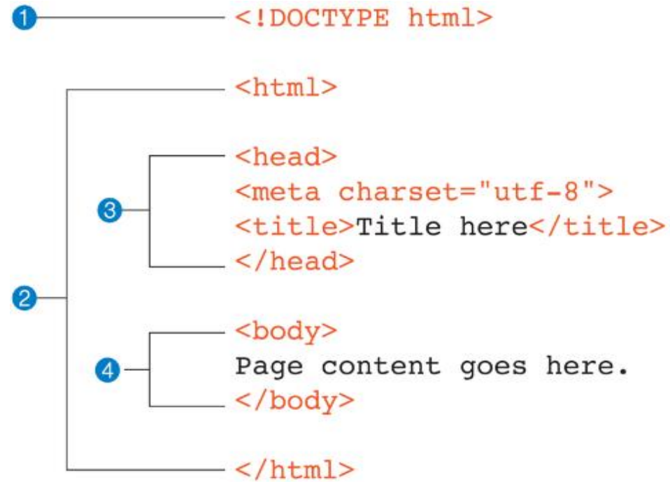
Figure 8 : Structure minimale d'un document html
