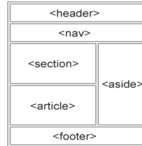
Figure 24 : Les éléments sémantiques [8]
