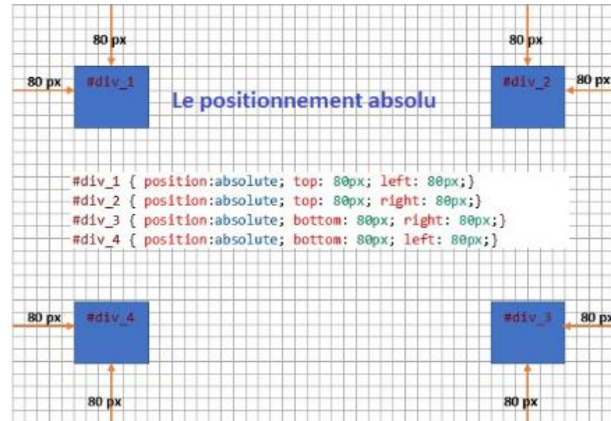
Figure 41: positionnement absolu en CSS
